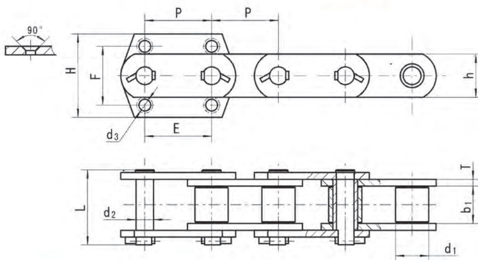
NSE 型 TYPE NSE
