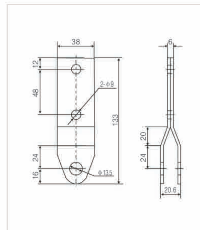
X348 "H" 型
