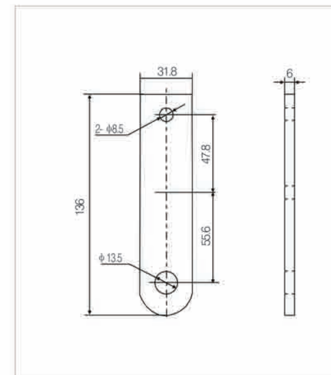
X348 "C" 型
