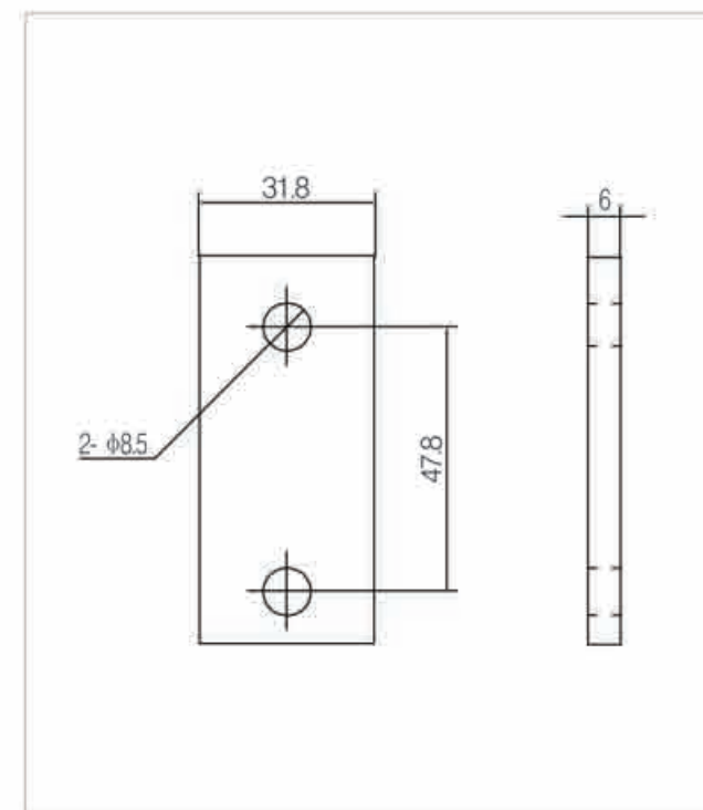
X348 "I" 型
