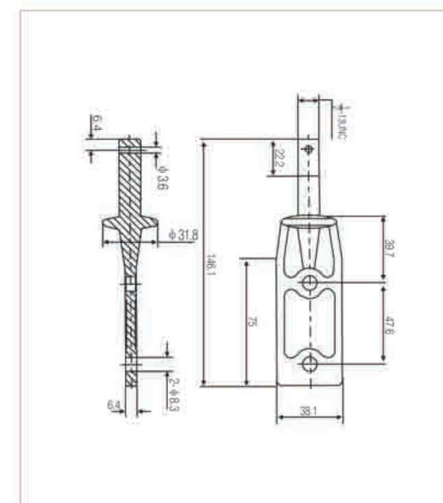
X348 "B" 型
